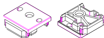
Уплотнительная колодка Арт.-№: 106.218 Цвет: белый
