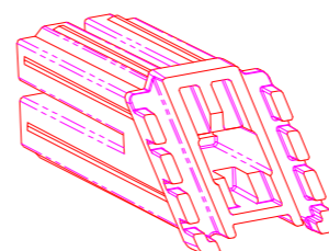
Сварной соединитель углов для 113.049.2 арт. 141.515
